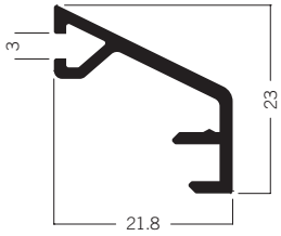
C 154 Glashalteprofil 22 × 23 mm 1.42 kg | 6000 mm
