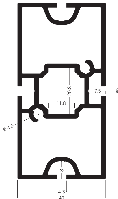
M 1025 Rechteckprofil 80 mm 10.22 kg | 5000 mm
