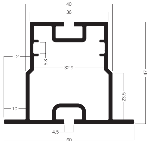
W 825* Rahmenprofil 60 mm Paneel (USA) 7.20 kg l 5000 mm
