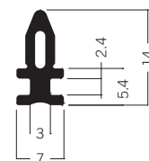
C 725 Verbindungsprofil 0.26 kg | 5950 mm
