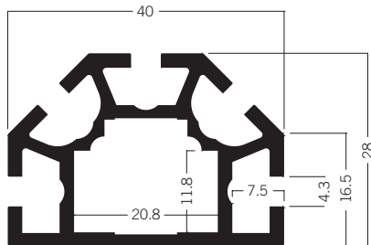
S 201 Stützenprofil 40 mm 4.25 kg | 5000 mm
