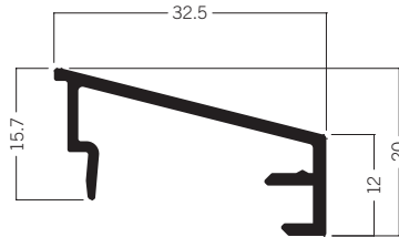
C 171 Horizontales Halteprofil 33 × 12 mm 1.64 kg | 6000 mm
