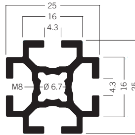
S 10* Quadratprofil 25 mm 3.08 kg | 5000 mm
