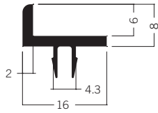
E 442 Auflageprofil 0.40 kg | 5000 mm
