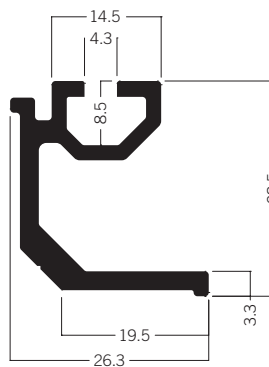
M 1326 Anschlussprofil Kubus 3.27 kg | 6000 mm
