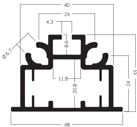
S 1610* Rahmenprofil 48 mm 6.48 kg l 6000 mm
