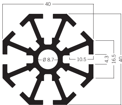
S 100 Stützenprofil 40 mm 6.80 kg | 5000 mm
