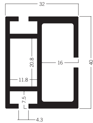
Z 2105 Zargenprofil 40 mm 5.56 kg | 5000 mm
