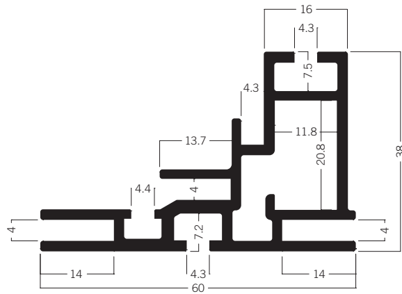
M 1910 Spannrahmenprofil für Leuchtrahmen 60 mm 7.62 kg | 6000 mm
