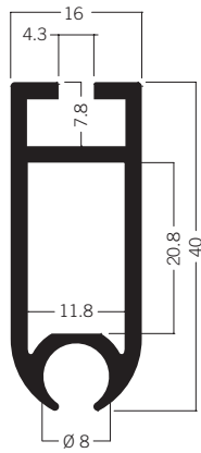
M 1354 Stoffhalteprofil 40 mm 3.18 kg | 5000 mm
