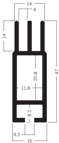
M 1504 Spannrahmenprofil Kubus 4.57 kg | 6000 mm
