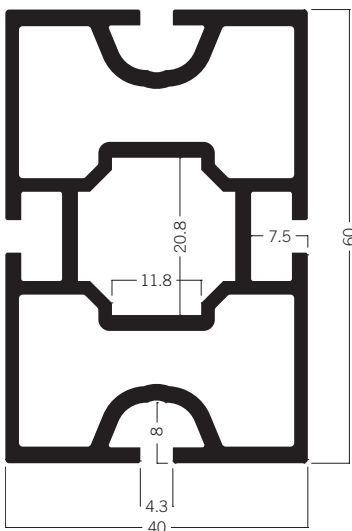
M 1081 Rechteckprofil 60 mm 8.94 kg | 5000 mm
