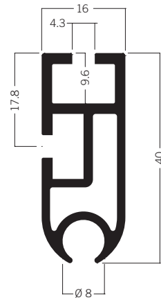
M 1356 Stoffhalteprofil 40 mm 3.20 kg | 5000 mm
