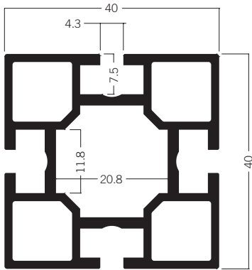
M 1000 Quadratprofil 40 mm 5.78 kg | 5000 mm
