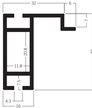
Z 4100 Zargenprofil 40 mm 4.14 kg | 5000 mm
