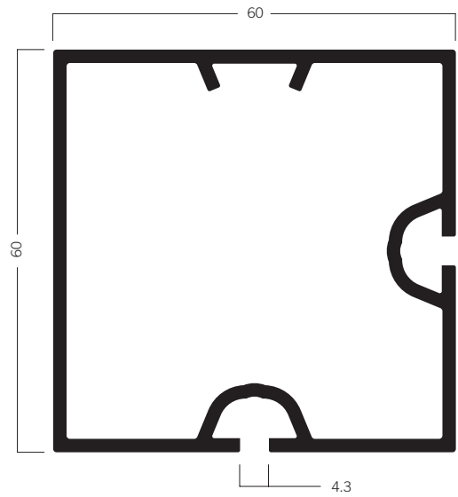
C 60-1007 Eckstützenprofil 60 × 60 mm 9.18 kg | 6000 mm
