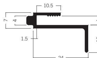
E 410 Schiebetür-Griffleistenprofil 0.50 kg | 5000 mm
