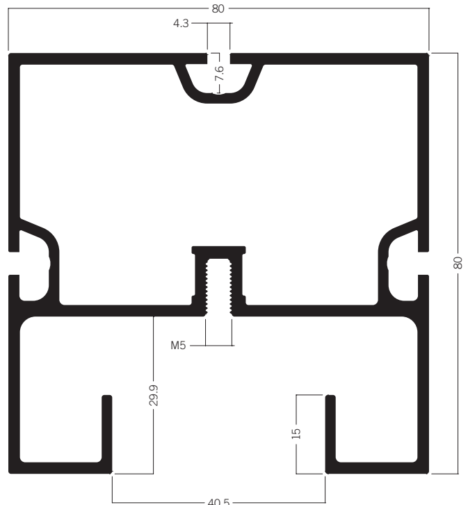
M 1059 Stromschienehalterprofil 80 mm 15.92 kg | 6000 mm
