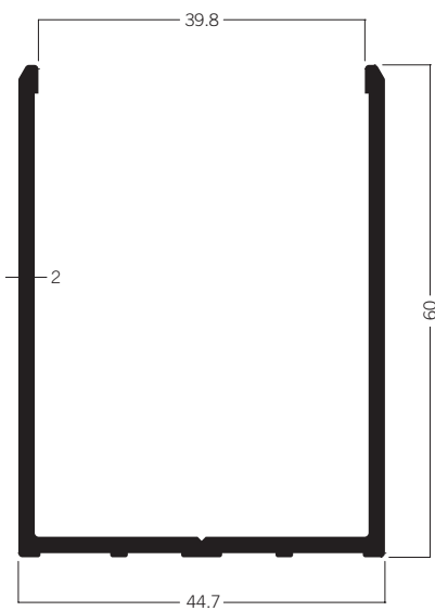
C 130 Boden U-Profil 45 × 60 mm 5.33 kg | 6000 mm
