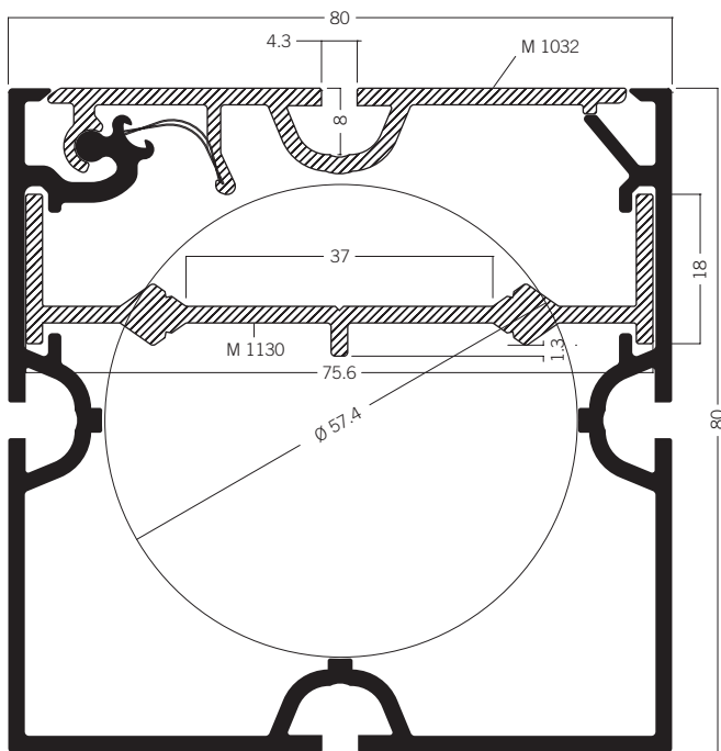
M 1022* Quadratprofil 80 mm 15.66 kg | 5000 mm
