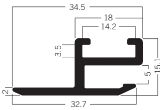
C 875 Rahmenprofil 34.5 × 15 mm 2.22 kg | 6000 mm
