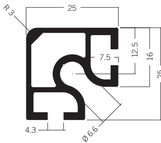
V 2000 Quadratprofil 25 mm 2.89 kg | 5000 mm
