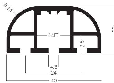
M 1606 Halbkreisprofil 40 mm 3.04 kg | 5000 mm
