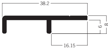
M 1562 Wandaufnahmeprofil oben 1.37 kg | 5000 mm
