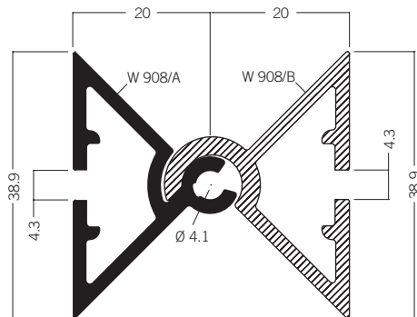
W 908 Scharnierprofil 5.60 kg | 5000 mm
