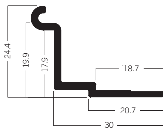
C 613 Auflageprofil 30 × 24 mm 1.82 kg | 6000 mm
