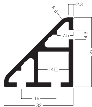
S 1303 Dreieckprofil 32 mm 3.19 kg | 5000 mm
