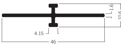
C 1415 Adaptionprofil Verglasung 1.58 kg | 6000 mm
