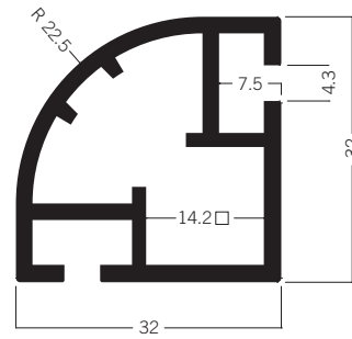
S 1100 Viertelkreisprofil 32 mm 4.06 kg | 5000 mm
