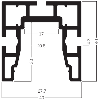
C 404* Deckenprofil LED (USA) 8.05 kg | 6000 mm
