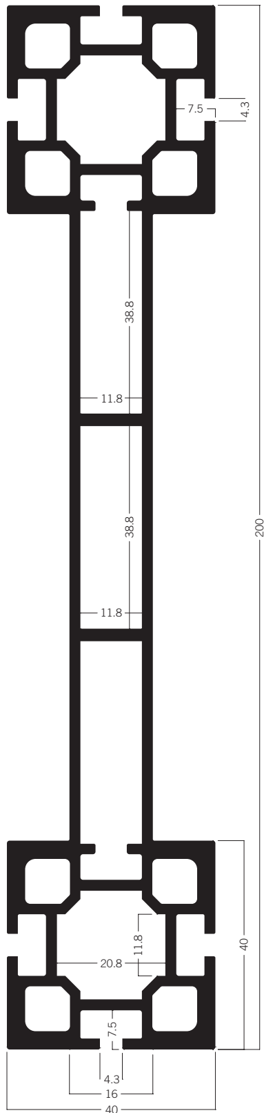
M 770 Trägerprofil 200 mm 35.53 kg | 7000 mm
