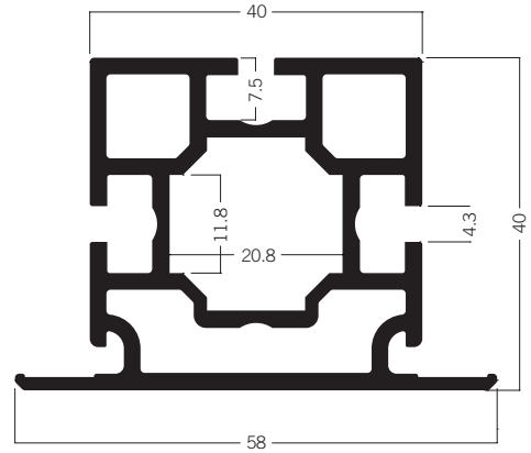
C 601 Profil 58 × 40 mm 8.69 kg | 6000 mm
