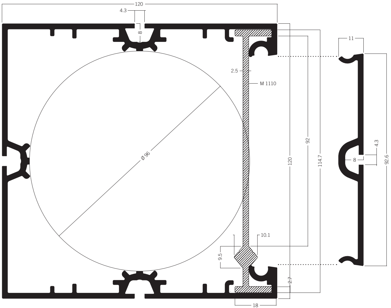
M 1041 Quadratprofil offen 120 mm 21.85 kg | 6000 mm
