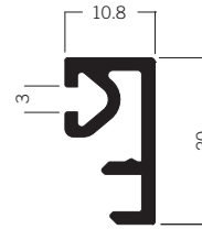
C 169 Glashalteprofil 11 × 20 mm 1.24 kg | 6000 mm
