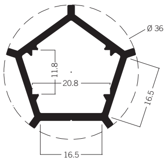
M 1980 Leuchtelementprofil 2.65 kg | 5000 mm
