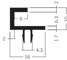
E 440 Glashalteprofil 0.47 kg | 5000 mm
