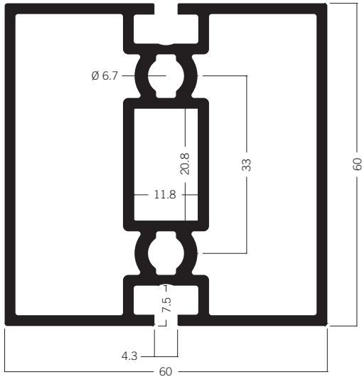
C 122 Zargenprofil 60 × 60 mm 13.03 kg | 6000 mm
