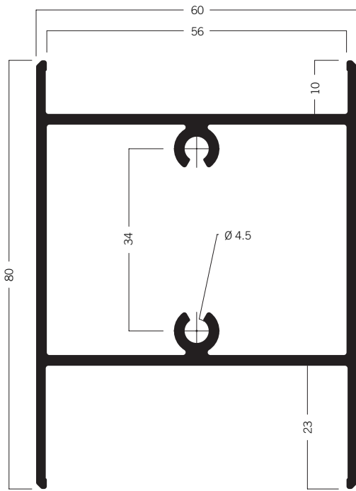
C 60-100 Zargenprofil 60 × 80 mm 9.88 kg | 6000 mm
