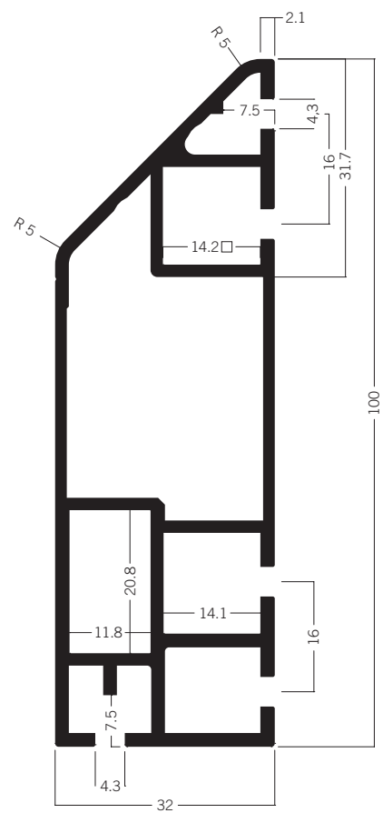
S 1310 Dreieckprofil 100 mm 9.28 kg | 5000 mm
