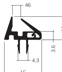
E 424 Glashalteprofil 0.45 kg | 5000 mm
