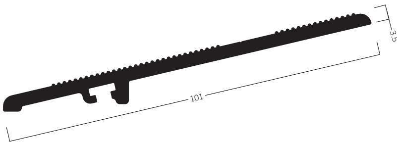
SO 640 Teppichleiste 5.48 kg | 5100 mm
