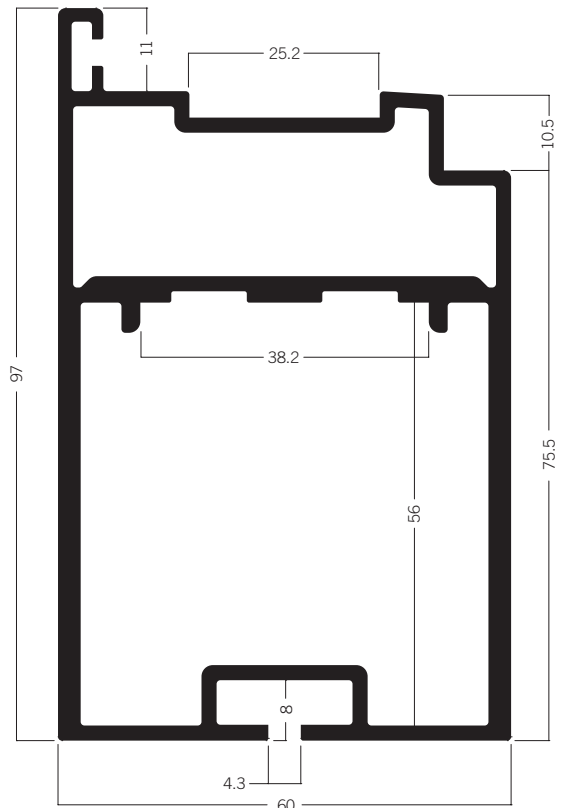
C 311 Doppeltürflügelprofil 60 × 97 mm 9.09 kg | 6000 mm
