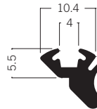
E 445 Klapperschutz 3.50 kg | 50000 mm
