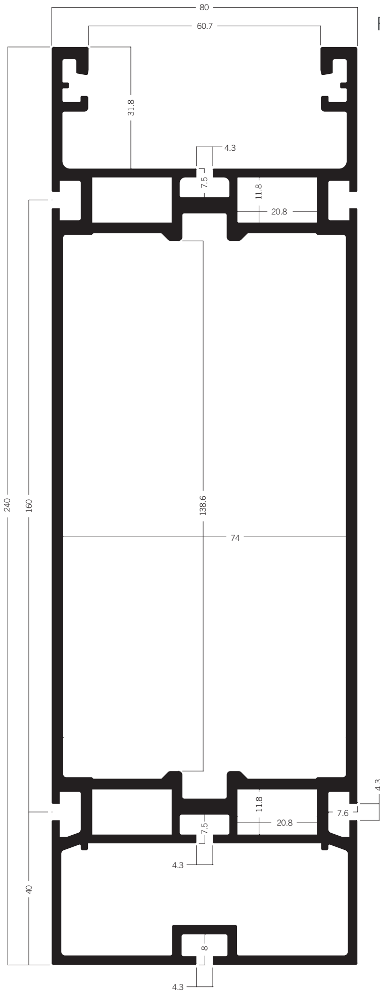
R 102 Rechteckträgerprofil 240 mm 53.23 kg | 6930 mm
