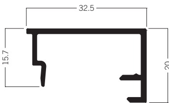
C 170 Vertikales Halteprofil 33 × 20 mm 1.38 kg | 6000 mm
