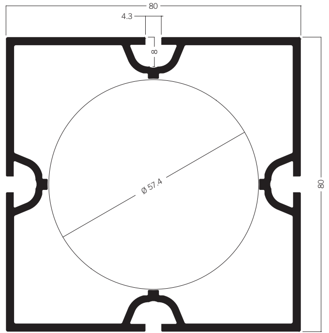
M 1020 Quadratprofil 80 mm 11.51 kg | 5000 mm
