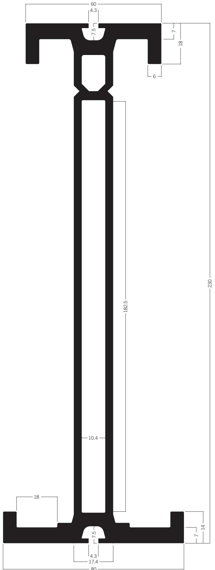
DFL 230 Trägerprofil 230 mm 53.24 kg | 7000 mm
