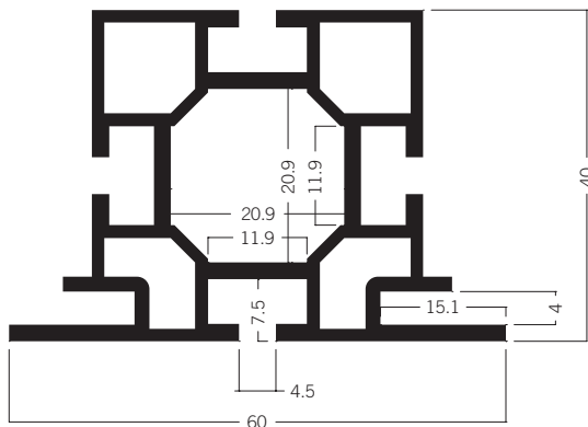
W 735R* Rahmenprofil 60 mm universal (USA) 9.20 kg | 6150 mm
