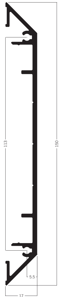
C 1327 Kabelkanalprofil 7.23 kg | 6000 mm
