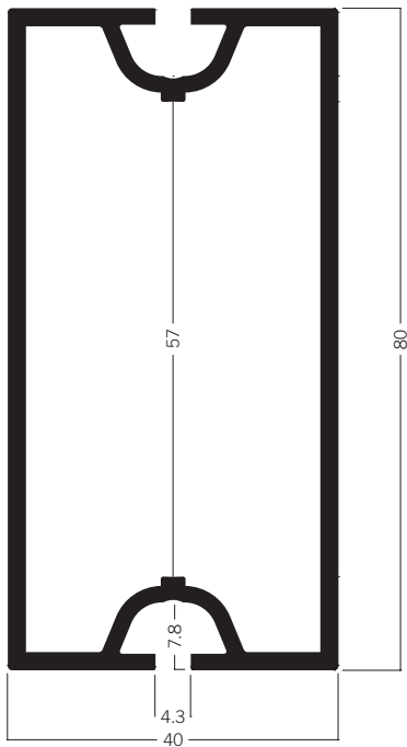
M 1043* Rechteckprofil 80 mm 5.61 kg | 5000 mm
