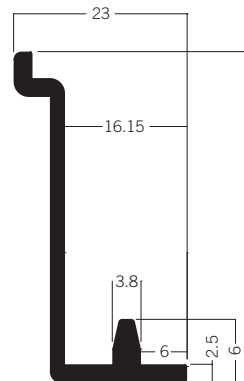
M 1581 Wandaufnahmeprofil unten 2.02 kg | 5000 mm
