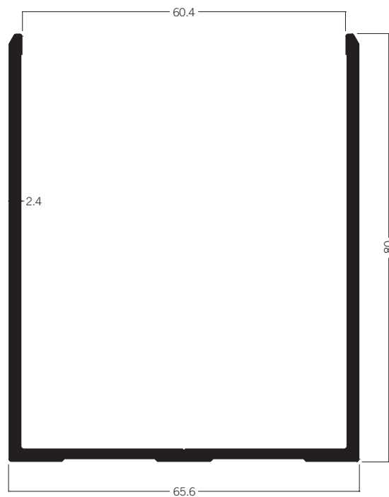
C 1005* Boden und Decken U-Profil 66 × 80 mm 8.47 kg | 6000 mm
