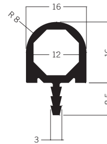
S 252 Gelenkprofil 16 mm 1.73 kg | 5000 mm
