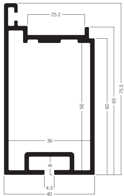
C 305 Fensterflügelprofil 40 × 75.5 mm 8.62 kg | 6000 mm
