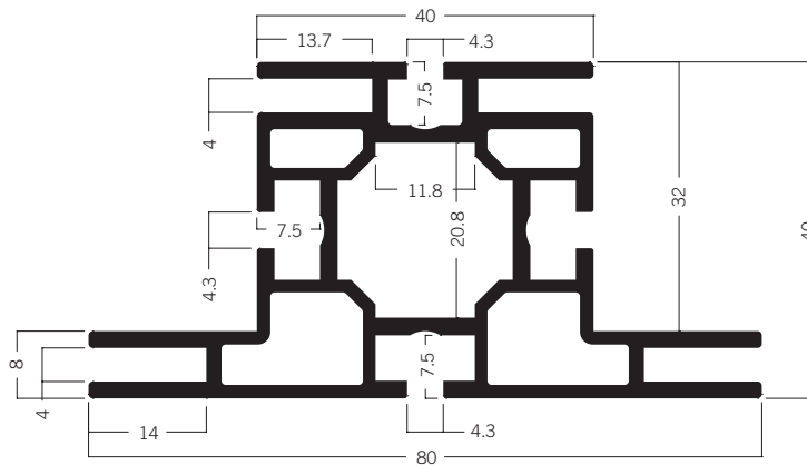
M 1304 Spannrahmenprofil 80 mm 10.15 kg | 6000 mm
