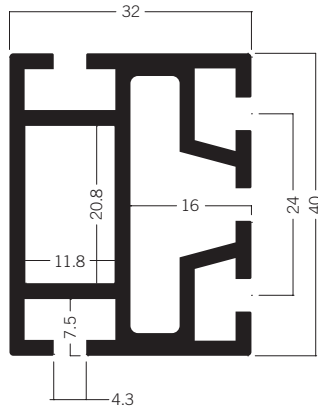
Z 2100 Zargenprofil 40 mm 5.99 kg | 5000 mm
