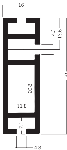
Z 464* Zargenprofil 50 mm 4.11 kg | 5000 mm
