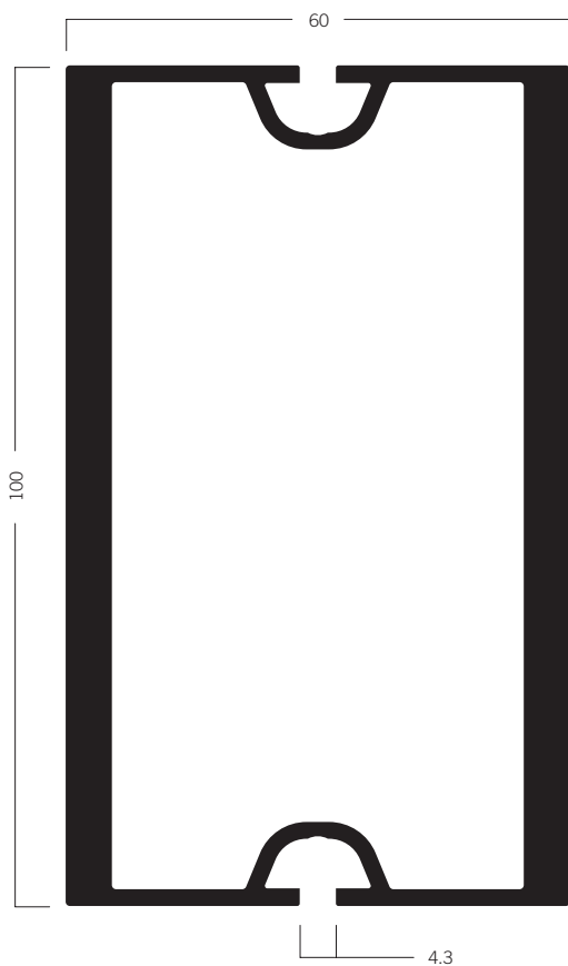
C 60-1029 Stützenprofil 60 × 100 mm 27.00 kg | 6000 mm
