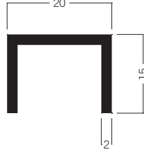
M 1312 U-Profil 1.56 kg | 6000 mm
