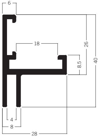
M 1302 Spannrahmenprofil 40 mm 3.49 kg | 6000 mm
