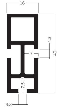
Z 4700 Rechteckprofil 40 mm 3.49 kg | 5000 mm
