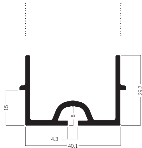
M 1155 Abdeckprofil für M 1059 3.46 kg | 5000 mm
