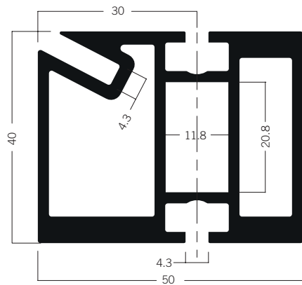
CO 730* Spannrahmenprofil 11.75 kg | 6100 mm
