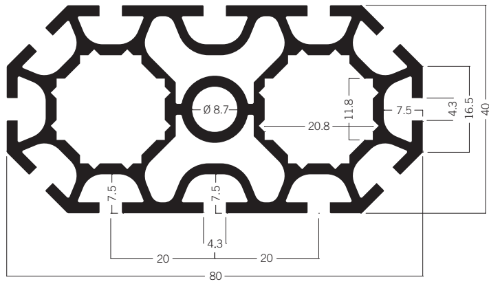
S 408 Stützenprofil 80 mm 12.64 kg | 5000 mm
