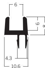
E 421 Glashalteprofil 0.41 kg | 5000 mm
