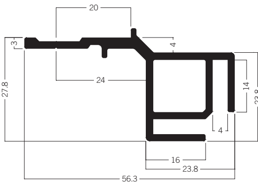
M 1322/I Spannrahmenprofil Inneneck 4.61 kg | 6000 mm
