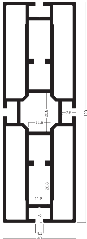
M 1031 Rechteckprofil 120 mm 18.07 kg | 6000 mm
