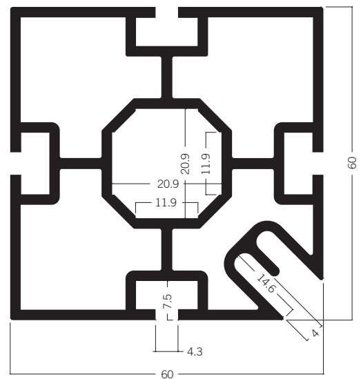
S 385R* Stützenprofil mit Kedernut (USA) 14.01 kg | 6150 mm
