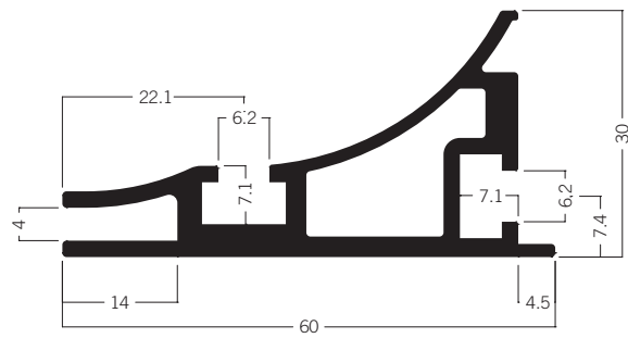
M 1920 Spannrahmenprofil für Leuchtrahmen 60 mm 6.07 kg | 6000 mm
