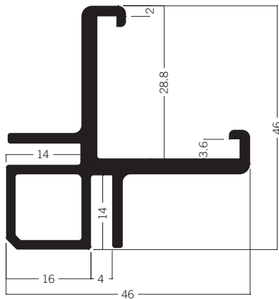
M 1332 Spannrahmenprofil Kubus 5.94 kg | 6000 mm
