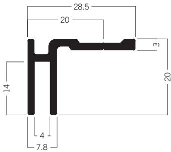
M 1322 Spannrahmenprofil 20 mm 2.03 kg | 6000 mm
