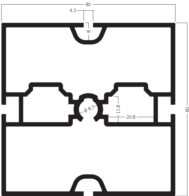
M 1018 Quadratprofil 80 mm 14.91 kg | 5000 mm
