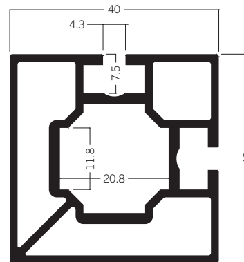
M 1007 Quadratprofil 40 mm 7.17 kg | 6000 mm
