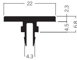
M 1844 Abdeckprofil 0.42 kg | 6000 mm
