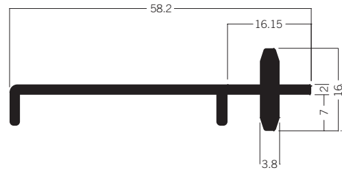
M 1577 Wandaufnahmeprofil Mitte 2.45 kg | 5000 mm
