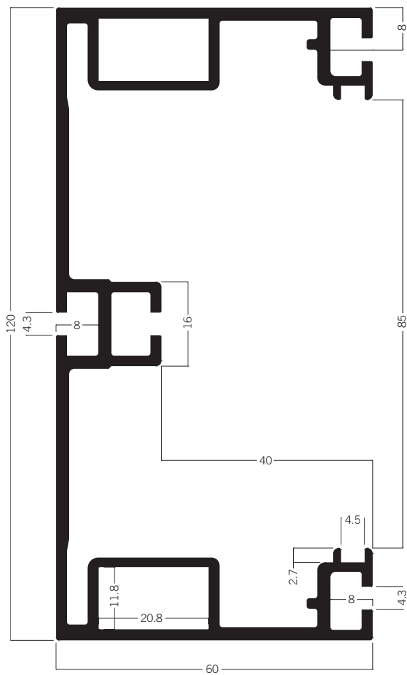
M 1060* Rechteckprofil offen 120 x 60 mm 5.61 kg | 5000 mm
