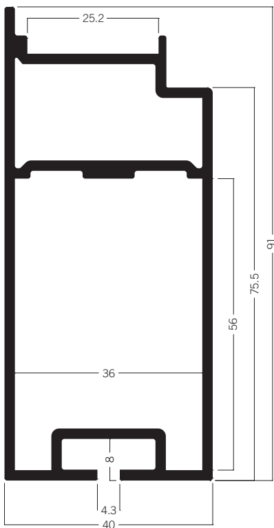
C 310 Doppeltürflügelprofil 40 × 91 mm 10.80 kg | 6000 mm
