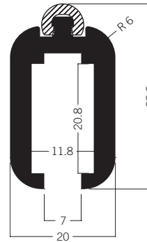
E 800 Garderobenstangenprofil 4.30 kg | 5000 mm
