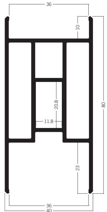
C 100 Zargenprofil 40 × 80 mm 9.98 kg | 6000 mm
