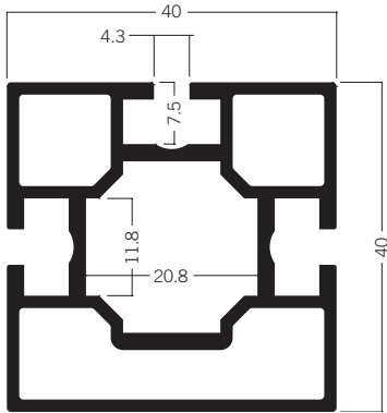
M 1005 Quadratprofil 40 mm 6.66 kg | 6000 mm
