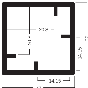
S 1123 Quadratprofil 32 mm 3.77 kg | 5000 mm
