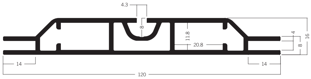
M 1901 Spannrahmenprofil für Leuchtrahmen 120 mm 9.77 kg | 6000 mm
