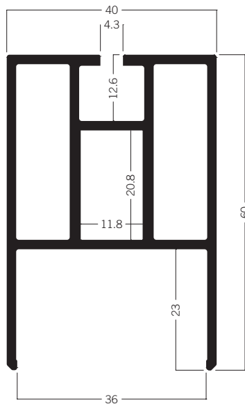
C 110 Zargenprofil 40 × 60 mm 7.57 kg | 6000 mm
