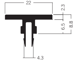
M 1846 Abdeckprofil 0.51 kg | 6000 mm
