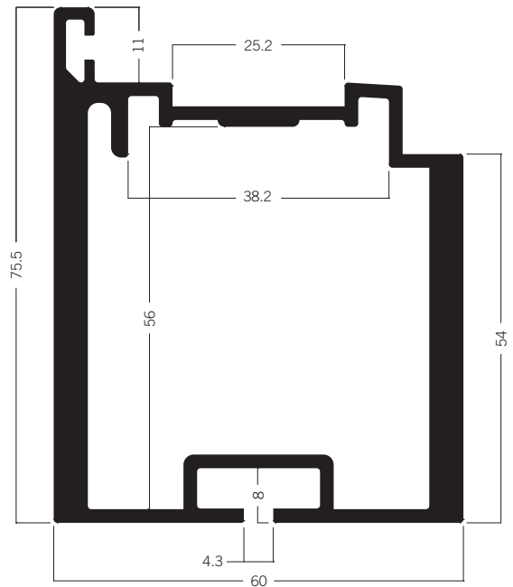
C 309 Türflügelprofil 60 × 75.5 mm 14.46 kg | 5500 mm
