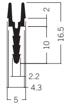
E 452 Verbindungsprofil 0.23 kg | 5000 mm
