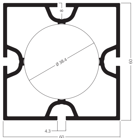
M 1010 Quadratprofil 60 mm 8.13 kg | 5000 mm
