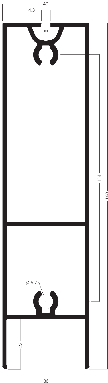
C 315 Türzargenprofil 40 × 160 mm 16.36 kg | 6000 mm
