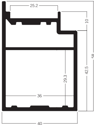
C 301 Türrahmenprofil 40 × 58 mm 7.54 kg | 6000 mm
