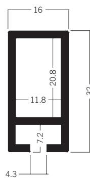
Z 308 Zargenprofil 32 mm 2.68 kg | 5000 mm
