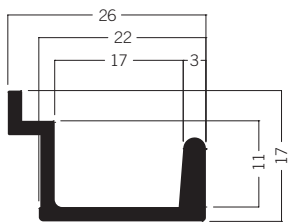
W 110* Adaptionprofil für vorgehängte Wand 1.47 kg | 5000 mm
