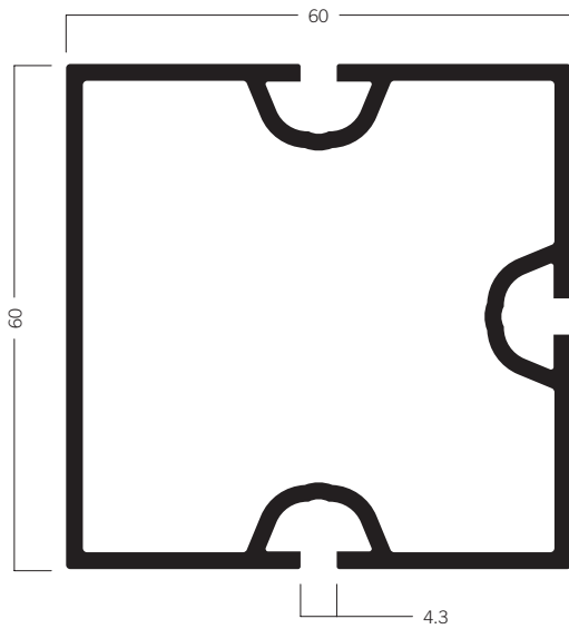
C 60-1005 Zargenprofil 60 × 60 mm 9.51 kg | 6000 mm
