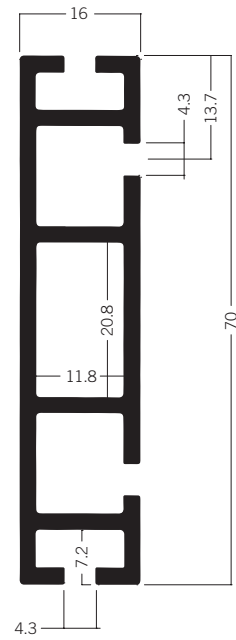
Z 164* Zargenprofil 70 mm 5.85 kg | 5000 mm
