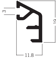
C 165 Glashalteprofil 12 × 19 mm 1.08 kg | 6000 mm
