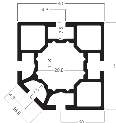
S 380 Stützenprofil 40 mm 5.97 kg | 5000 mm
