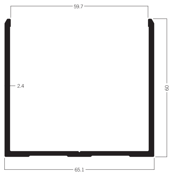
C 60-130 U-Profil 65 × 60 mm 6.90 kg | 6000 mm
