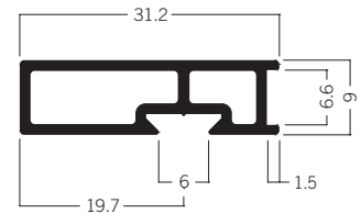
C 722 Halteprofil 31 × 9 mm 1.83 kg | 6000 mm
