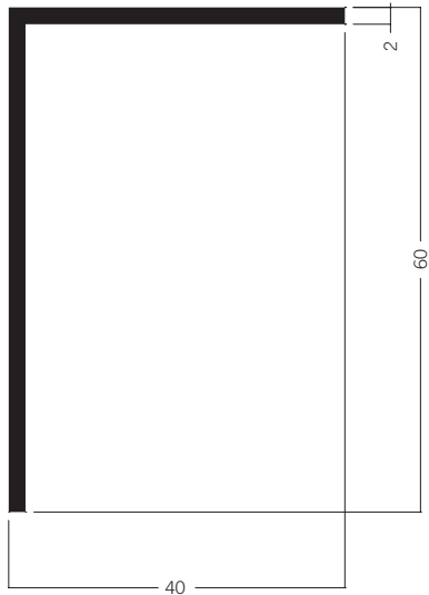
SO 500 Sockelwinkel 2.52 kg | 5000 mm
