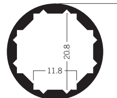
M 1208 Rundprofil 26.3 mm 2.17 kg | 5000 mm
