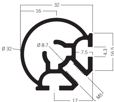
S 1200 Viertelkreisprofil 32 mm 3.78 kg | 5000 mm
