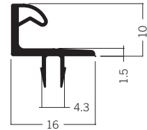
E 430 Türanschlagprofil 0.37 kg | 5000 mm
