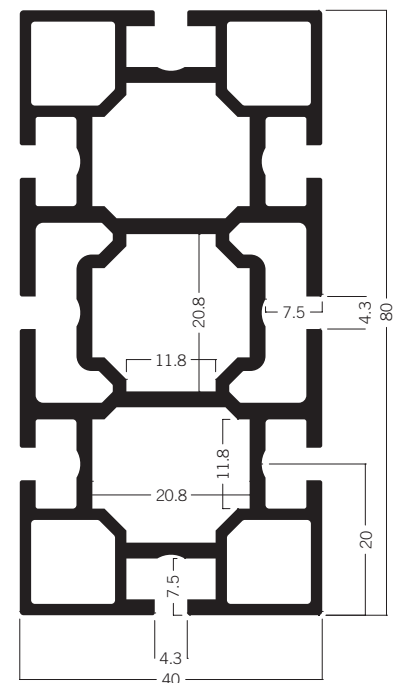
M 1092 Rechteckprofil 80 mm 14.60 kg | 6000 mm
