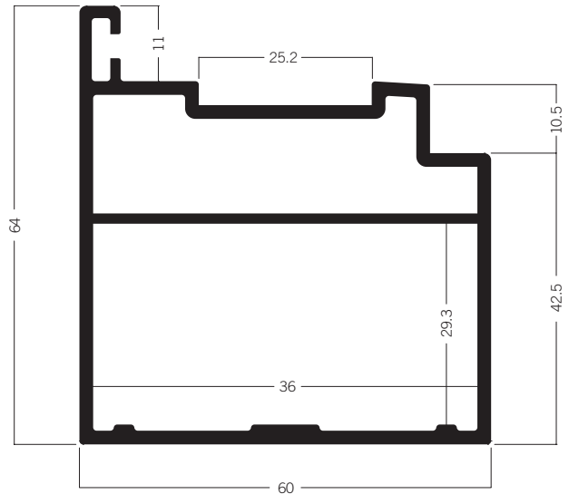
C 302 Türrahmenprofil 60 × 64 mm 9.51 kg | 6000 mm
