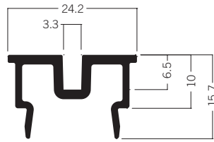
C 153 Distanzprofil 24 × 16 mm 1.69 kg | 6000 mm
