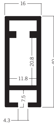
Z 4401 Zargenprofil 40 mm 3.38 kg | 5000 mm
