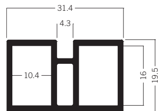
C 1220 Rahmenprofil 20 × 31 mm 3.42 kg | 6000 mm
