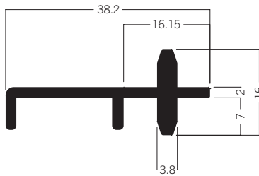
M 1567 Wandaufnahmeprofil Mitte 2.04 kg | 5000 mm
