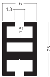
M 1602 Zargenprofil 25 mm 2.72 kg | 5000 mm
