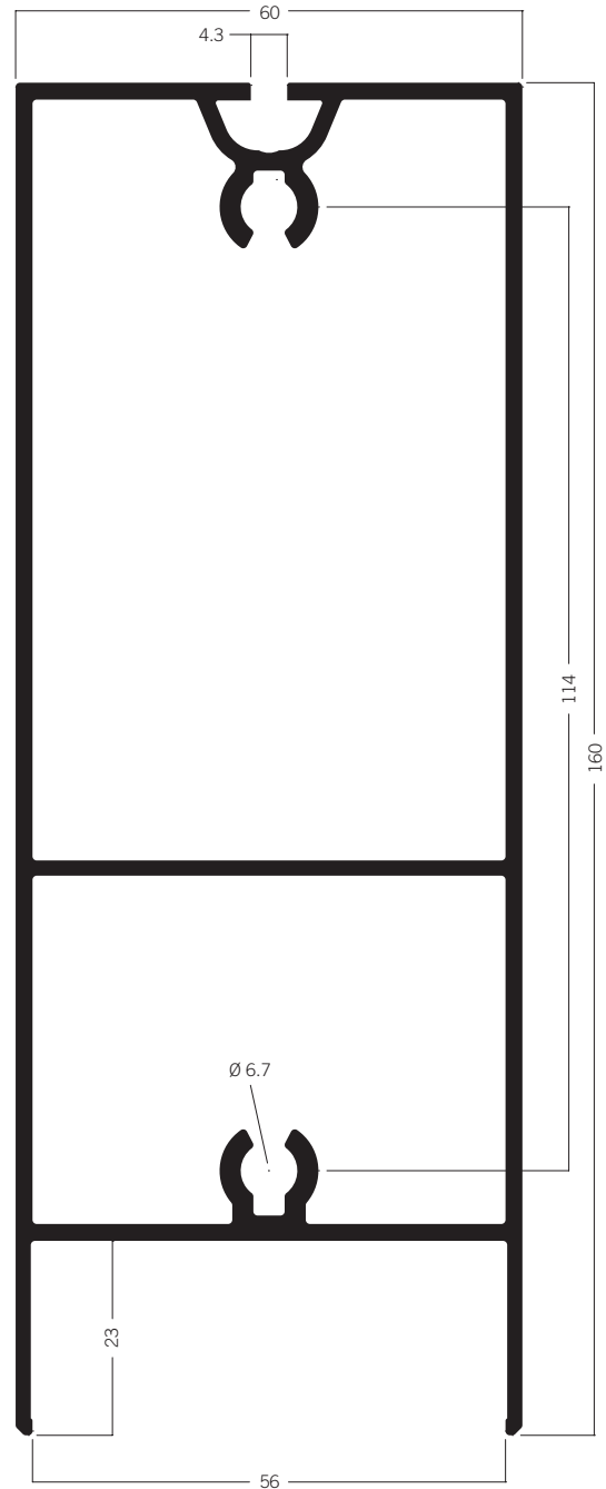
C 316 Türzargenprofil 60 × 160 mm 18.12 kg | 6000 mm
