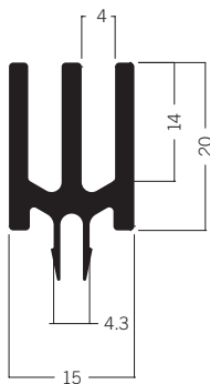
M 1319 Spannrahmenprofil 20 mm 1.46 kg | 6000 mm
