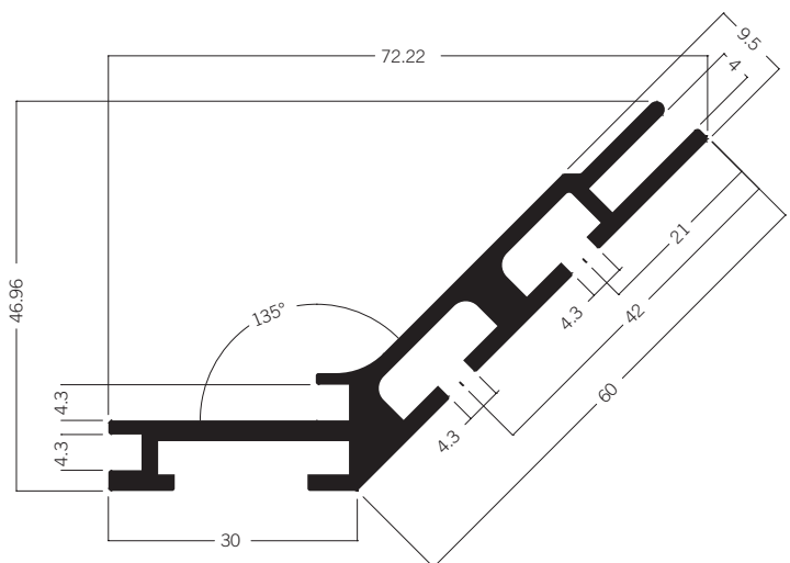
M 1301 Spannrahmenprofil 135° 6.55 kg | 6000 mm
