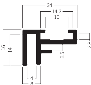
M 1607 Spannrahmenprofil 16 mm 1.91 kg | 6000 mm
