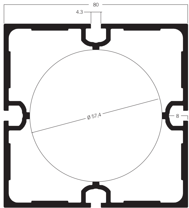
U 1020 Quadratprofil 80 mm 15.50 kg | 6000 mm
