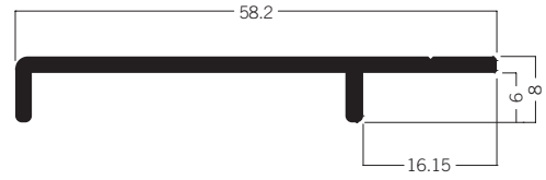
M 1572 Wandaufnahmeprofil oben 1.77 kg | 5000 mm
