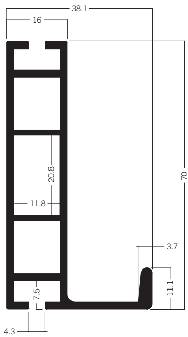
W 103 Zargenprofil 70 mm 6.51 kg | 5000 mm
