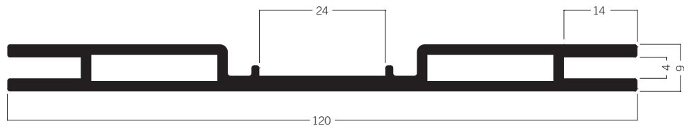
M 1330 Spannrahmenprofil 120 mm 8.28 kg | 6000 mm
