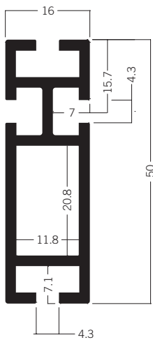
Z 460 Zargenprofil 50 mm 3.96 kg | 5000 mm
