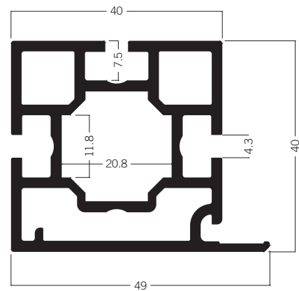
C 701 Profil 49 × 40 mm 8.88 kg | 6000 mm
