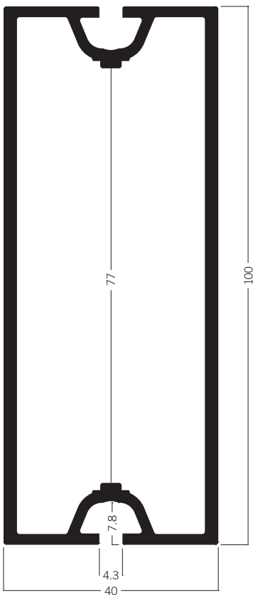
M 1029 Rechteckprofil 100 mm 11.88 kg | 6000 mm
