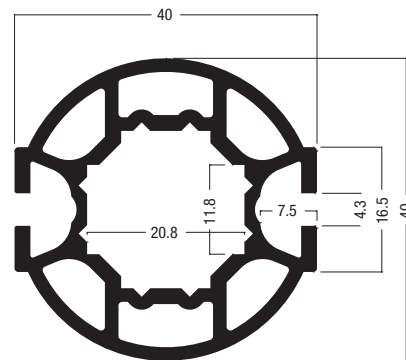
M 1208 Rundprofil 26.3 mm 2.17 kg | 5000 mm
