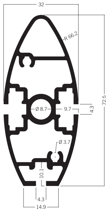
S 6105 Ovalprofil 32 x 72.5 mm 7.65 kg l 5000 mm
