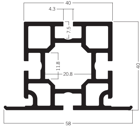
C 606 Profil 58 × 40 mm 9.50 kg | 6000 mm
