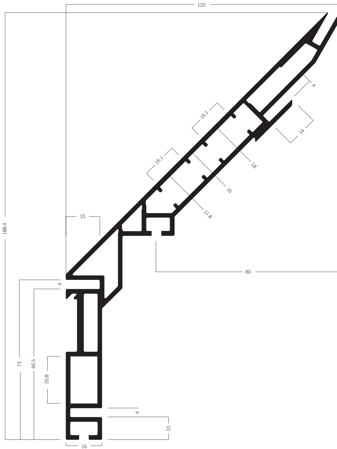
U 1063 Spannrahmenprofil 120 mm 21.51 kg | 6000 mm
