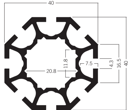
S 108 Stützenprofil 40 mm 5.35 kg | 5000 mm
