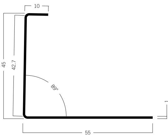
C 670 Deckenprofil 0.56 kg | 2400 mm
