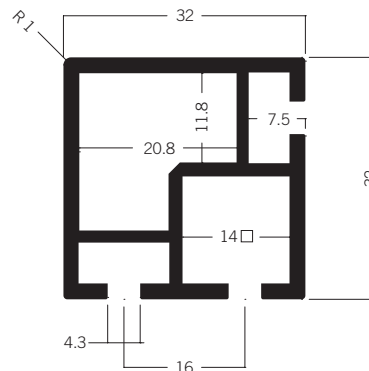
S 1125 Quadratprofil 32 mm 4.03 kg | 5000 mm
