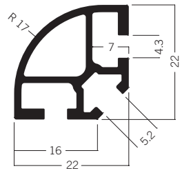
M 1620 Viertelkreisprofil 22 mm 1.80 kg | 5000 mm
