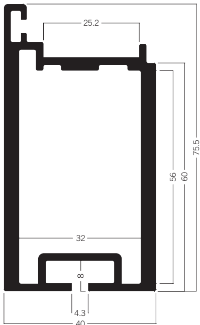
C 308 Türflügelprofil 40 × 75.5 mm 11.45 kg | 5500 mm
