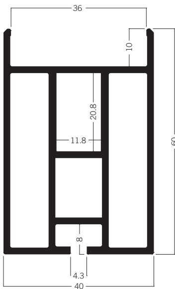
C 105 Zargenprofil 40 × 60 mm 9.26 kg | 6000 mm
