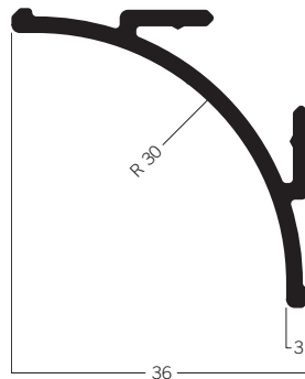
C 1301 Hohlkehlenprofil 36 × 36 mm 2.62 kg | 6000 mm
