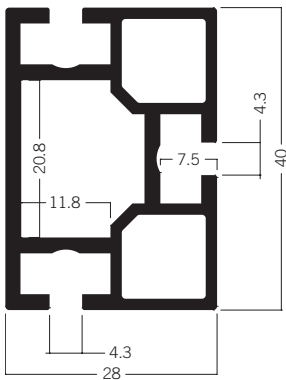
M 1069 Rechteckprofil 40 mm 5.71 kg | 6000 mm
