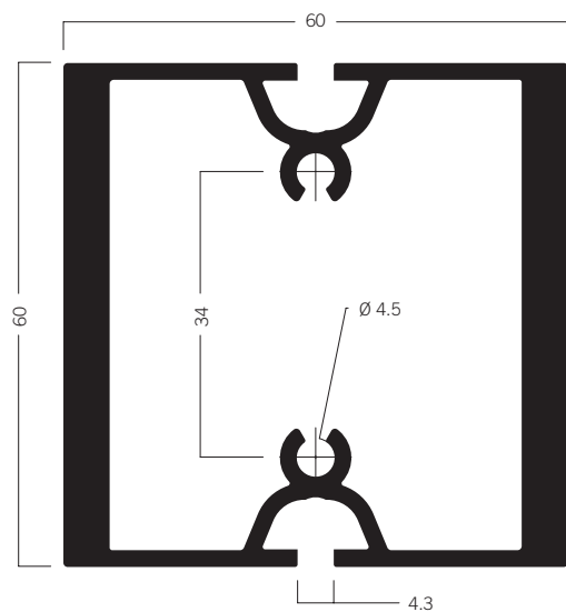
C 60-125 Stützenprofil 60 × 60 mm 16.25 kg | 6000 mm
