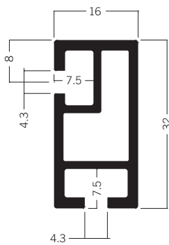
Z 307 Zargenprofil 32 mm 2.53 kg | 5000 mm
