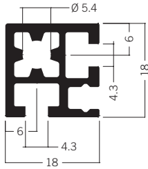
M 1618 Quadratprofil 18 mm 1.99 kg | 5000 mm
