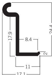
C 612 Auflageprofil 17 × 24 mm 1.11 kg | 6000 mm
