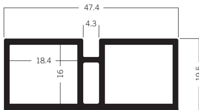
C 1210 Rahmenprofil für Türverglasung 4.33 kg | 6000 mm
