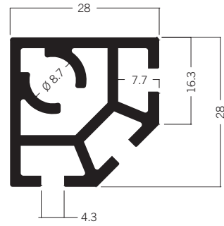
S 308 Stützenprofil 28 m 4.14 kg | 5000 mm
