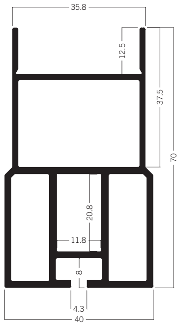
C 115 Zargenprofil 40 × 70 mm 9.03 kg | 6000 mm
