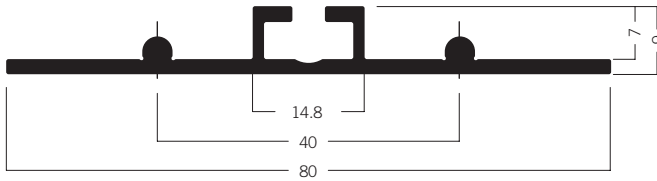
WP 830 Abdeckprofil für Profil WP 860 3.58 kg | 6060 mm
