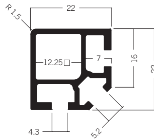
M 1625 Quadratprofil 22 mm 2.15 kg | 5000 mm
