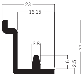
M 1571 Wandaufnahmeprofil unten 1.62 kg | 5000 mm
