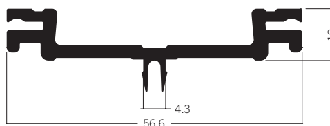
C 159 Adapterprofil 10 × 57 mm 2.04 kg | 6000 mm
