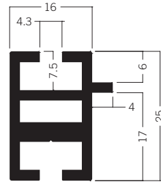
M 1603* Zargenprofil 25 mm 2.74 kg | 5000 mm
