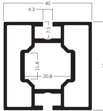
M 1002 Quadratprofil 40 mm 5.55 kg | 5000 mm
