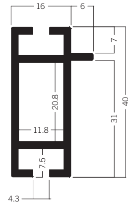
Z 4300 Zargenprofil 40 mm 3.54 kg | 5000 mm
