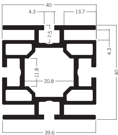
M 1305 Spannrahmenprofil 40 mm 8.23 kg | 6000 mm
