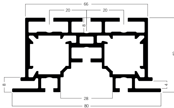
WP 860 Spannrahmenprofil 80 mm 12.99 kg | 6060 mm
