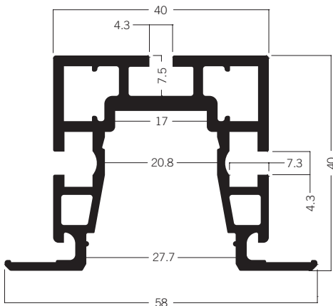
C 608 Deckenprofil LED 7.32 kg | 6000 mm
