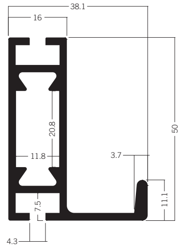
W 101 Zargenprofil 50 mm 5.56 kg | 5000 mm
