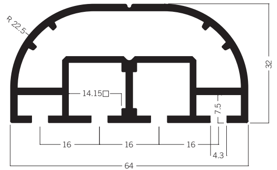
S 1106 Halbkreisprofil 64 mm 6.98 kg | 5000 mm
