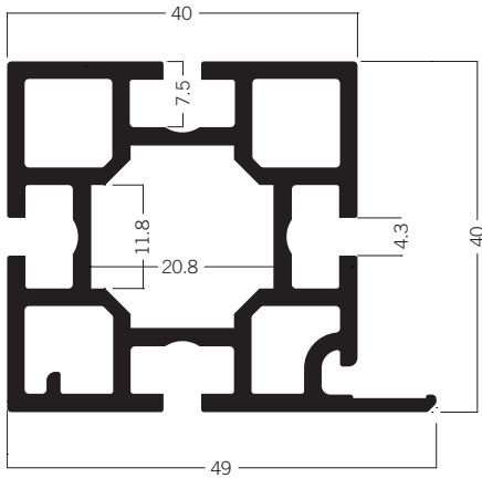
C 604 Profil 49 × 40 mm 9.15 kg | 6000 mm
