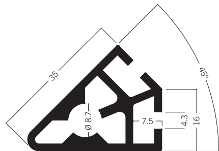
S 302 Stützenprofil 45° 4.03 kg | 5000 mm
