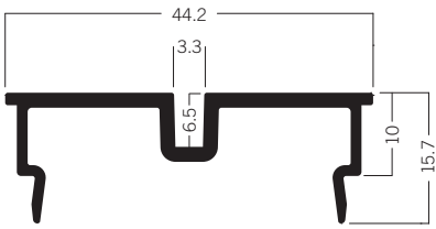
C 151 Distanzprofil 44 × 16 mm 2.28 kg | 6000 mm
