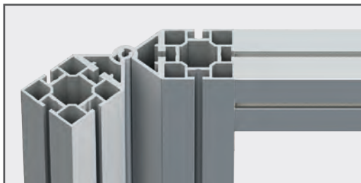
Winkel zwischen 90° und 180° können frei mit dem Scharnierprofil W 908 reali- siert werden.
