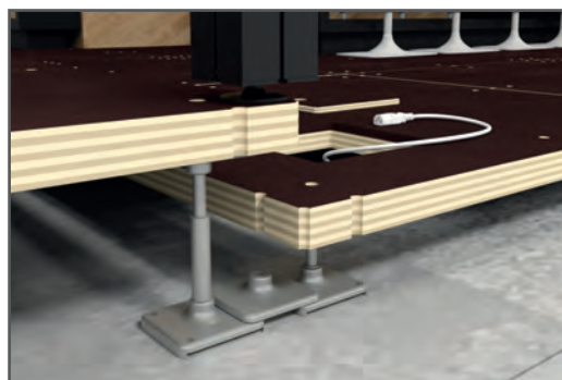
Das Doppelbodensystem OCTAfloor ermöglicht effizientes Leitung- und Kabelverlegen ebenso wie Podestbau.
