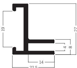
M 1309 Spannrahmenprofil für Kleinformate bis 841 × 1189 mm (DIN A0), 22,5 mm 2,53 kg | 6000 mm
