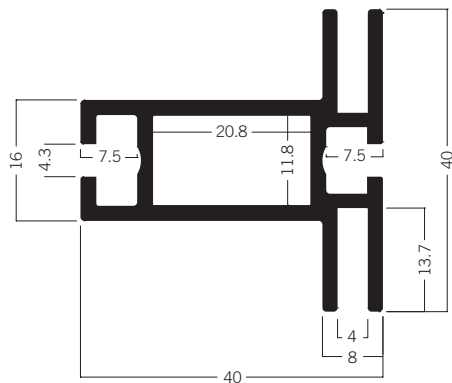
M 1307 Spannrahmenprofil für beidseitige Stoffbefestigung 40 mm 5,39 kg | 6000 mm
