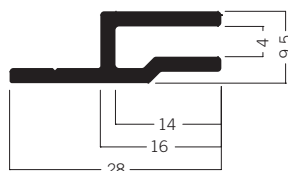
M 1614 Spannrahmenprofil 28 mm 1,54 kg | 6000 mm
