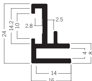
M 1607 Spannrahmenprofil für Kleinformate bis 594 × 841 mm (DIN A1), 16 mm 1,91 kg | 6000 mm
