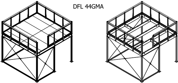
Bodenplatten oben für DFL 44GMA
