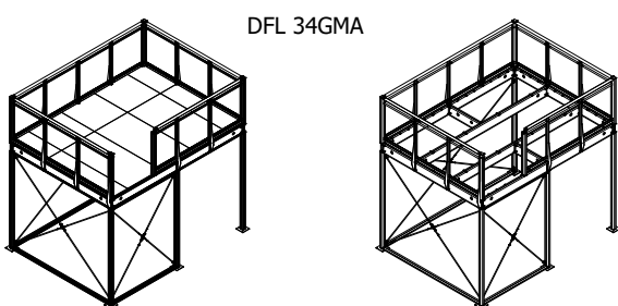
Bodenplatten oben für DFL 34GMA
