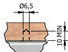
Detail C ( 1 : 2 )
