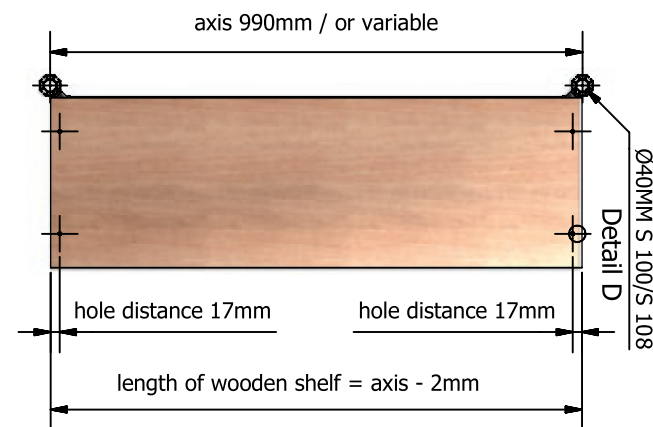
Detail D ( 1 : 2 )
