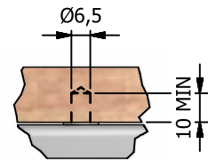
Detail E ( 1 : 2 )
