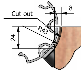
Detail E ( 1 : 2 )
