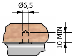
Detail A ( 1 : 2 )
