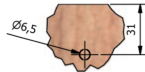
Detail D ( 1 : 2 )
