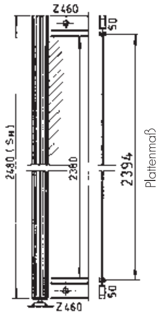
① S_H - 86 = Plattenhöhe
