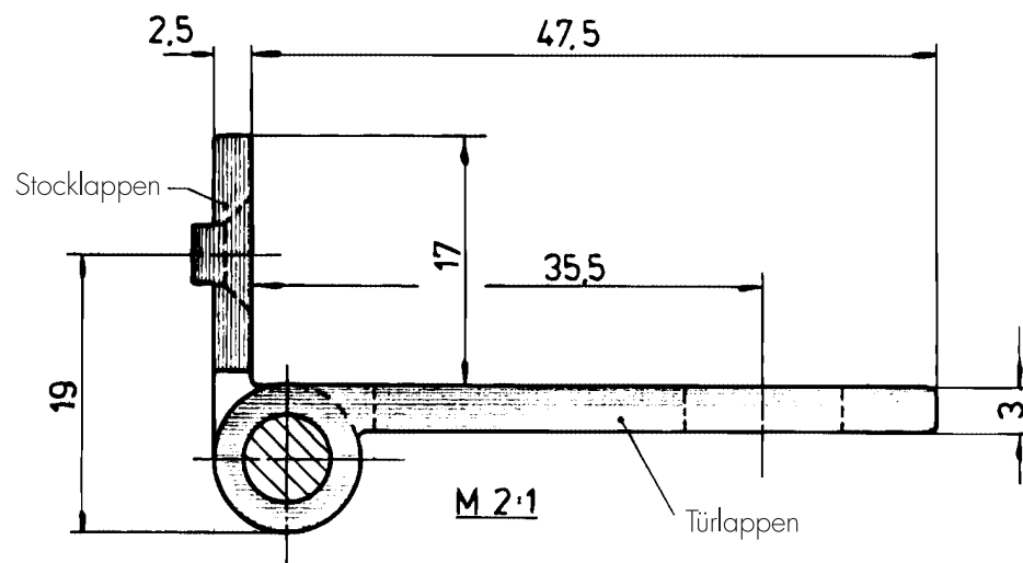
Detaildarstellung E 290
