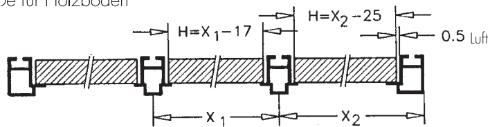
Maße für Holzböden
