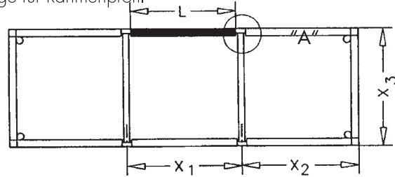
Maße für Glas-Tischplatten
