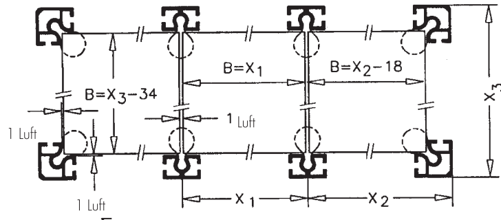
Maße für Holzböden
