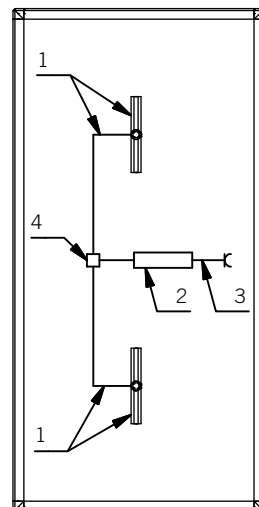
Kubus 2 Leuchtelemente
