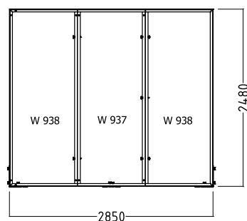
Aufbauvariante 3 Rahmen
