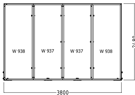
maximale Bauweise
