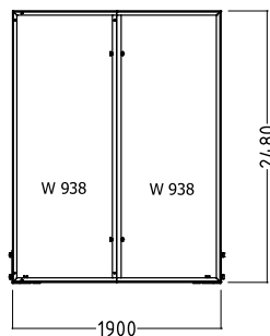
Aufbauvariante 2 Rahmen
