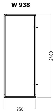
Rahmenelement Außen
