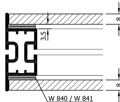
octawall 60 Standard Paneel: 8mm Haken-Flauschband: 3.5mm
