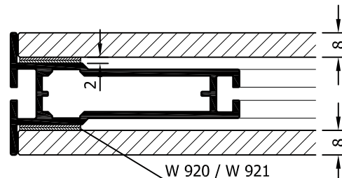
octawall 40 Standard Paneel: 8mm Haken-Flauschband: 2mm
