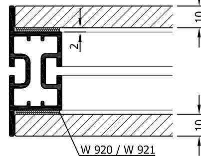
octawall 60 Variante 1 Paneel: 10mm Haken-Flauschband: 2mm
